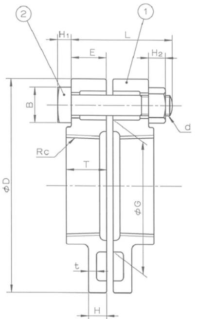
断面X-X
