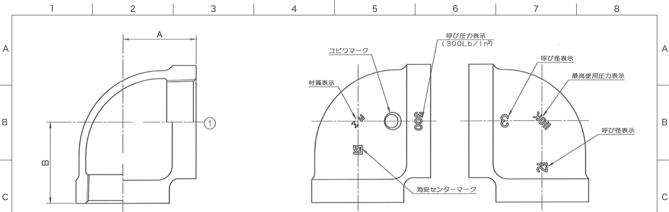
マーク配置図(例: 3×2½)
